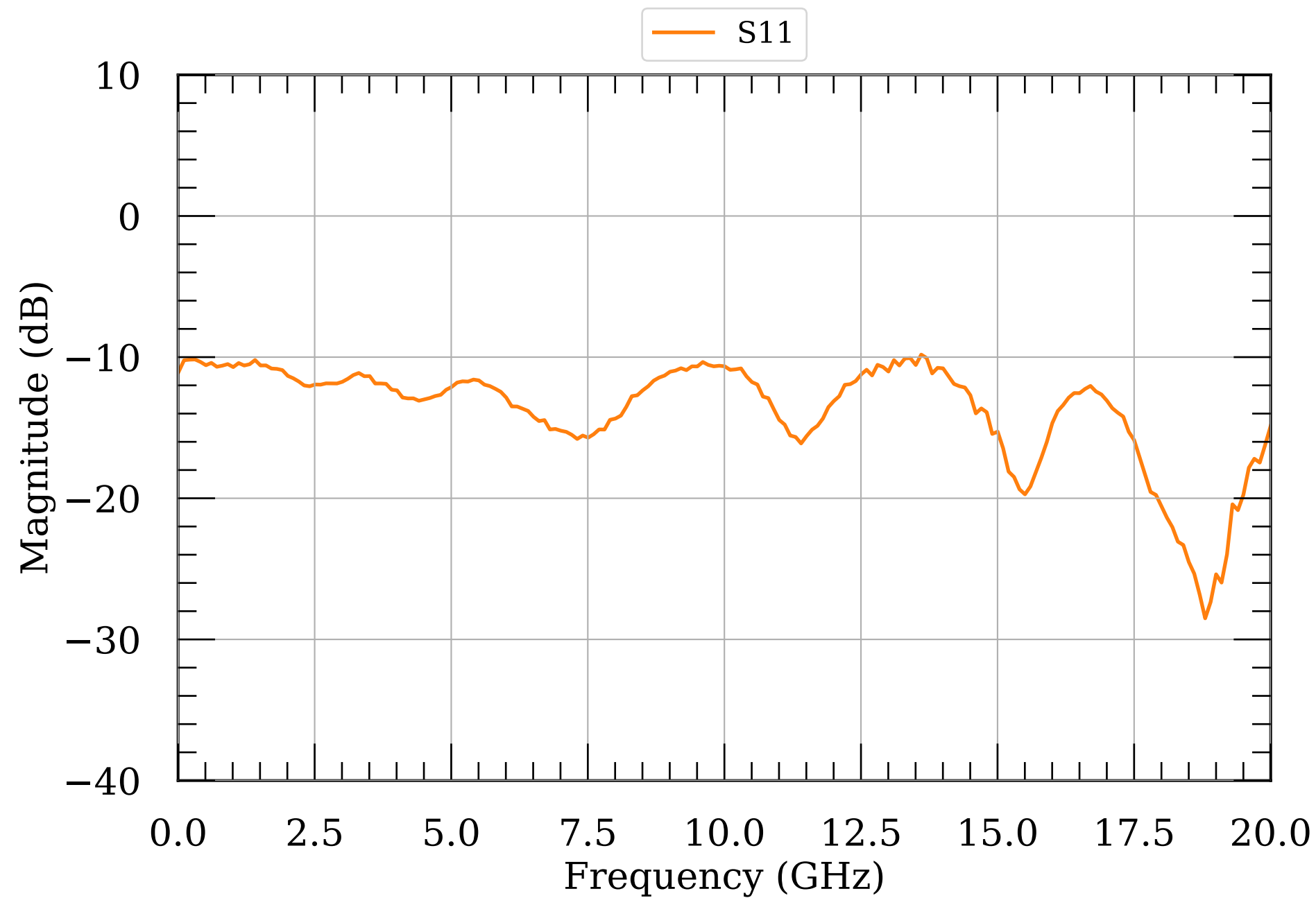
LNA S-params module038
